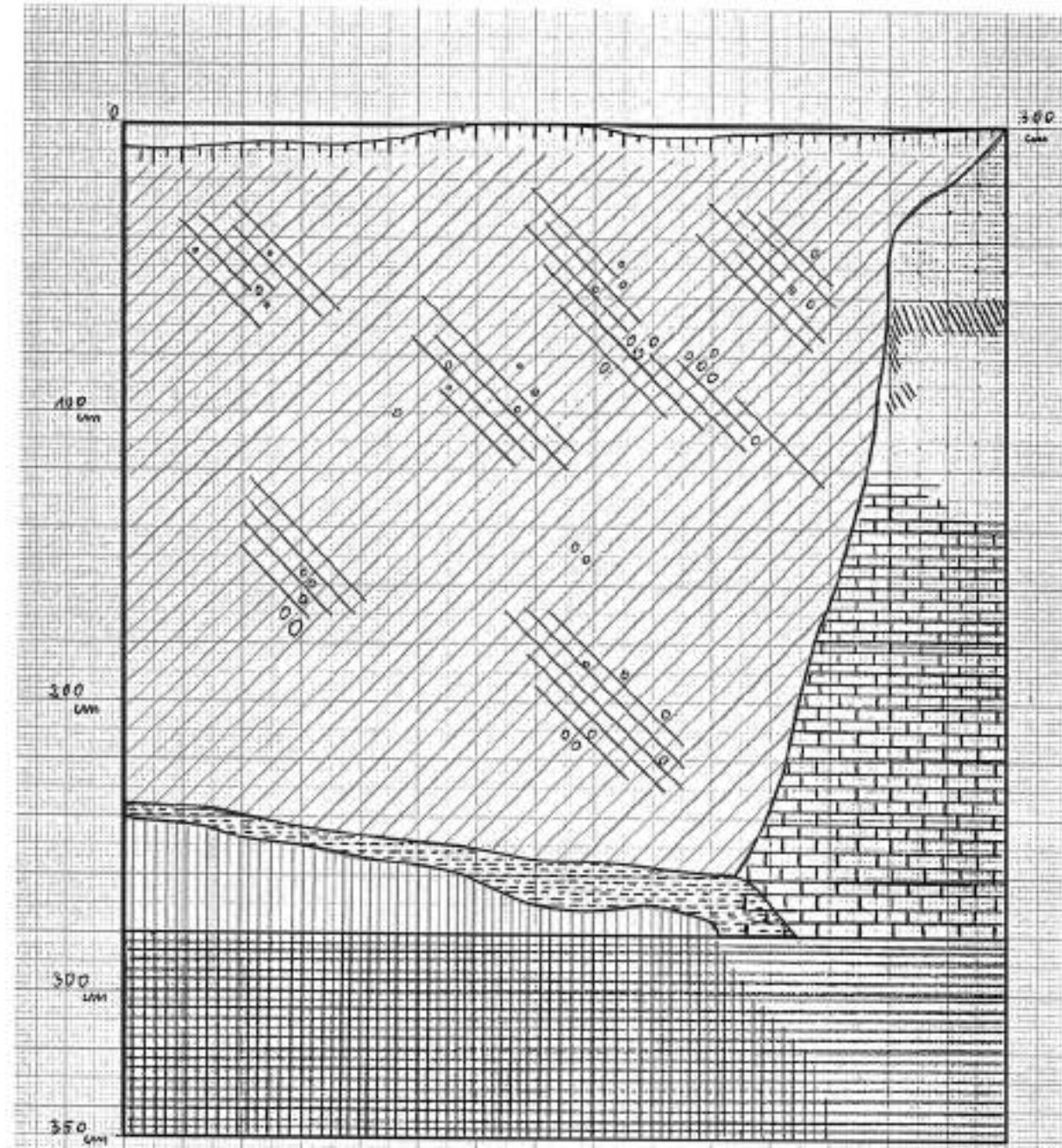
MIEDNOJE - JAMOK OBL. TVERSKA REP. ROSJA MIEJSCE POCHÓNKÓW POLSKICH STREFA "C" PROFIL "W" DOŁU ŚMIERCI NR 20 SKALA 1:20
