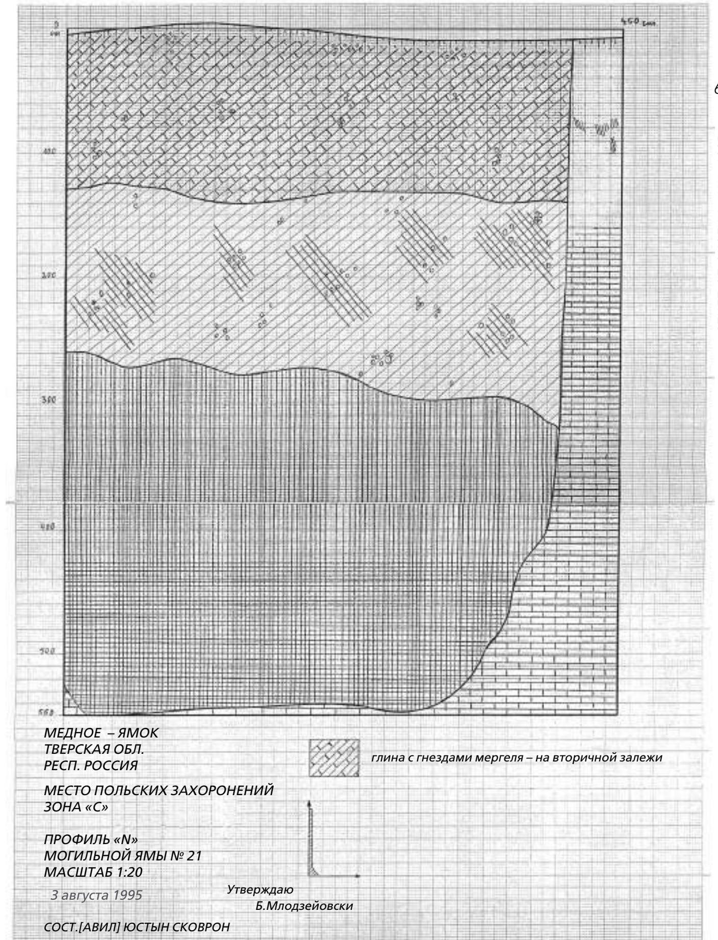
[Геологический профиль могильной ямы № 21. Условные обозначения объяснены на последней странице тома III отчета (см. ниже с. 650)]
