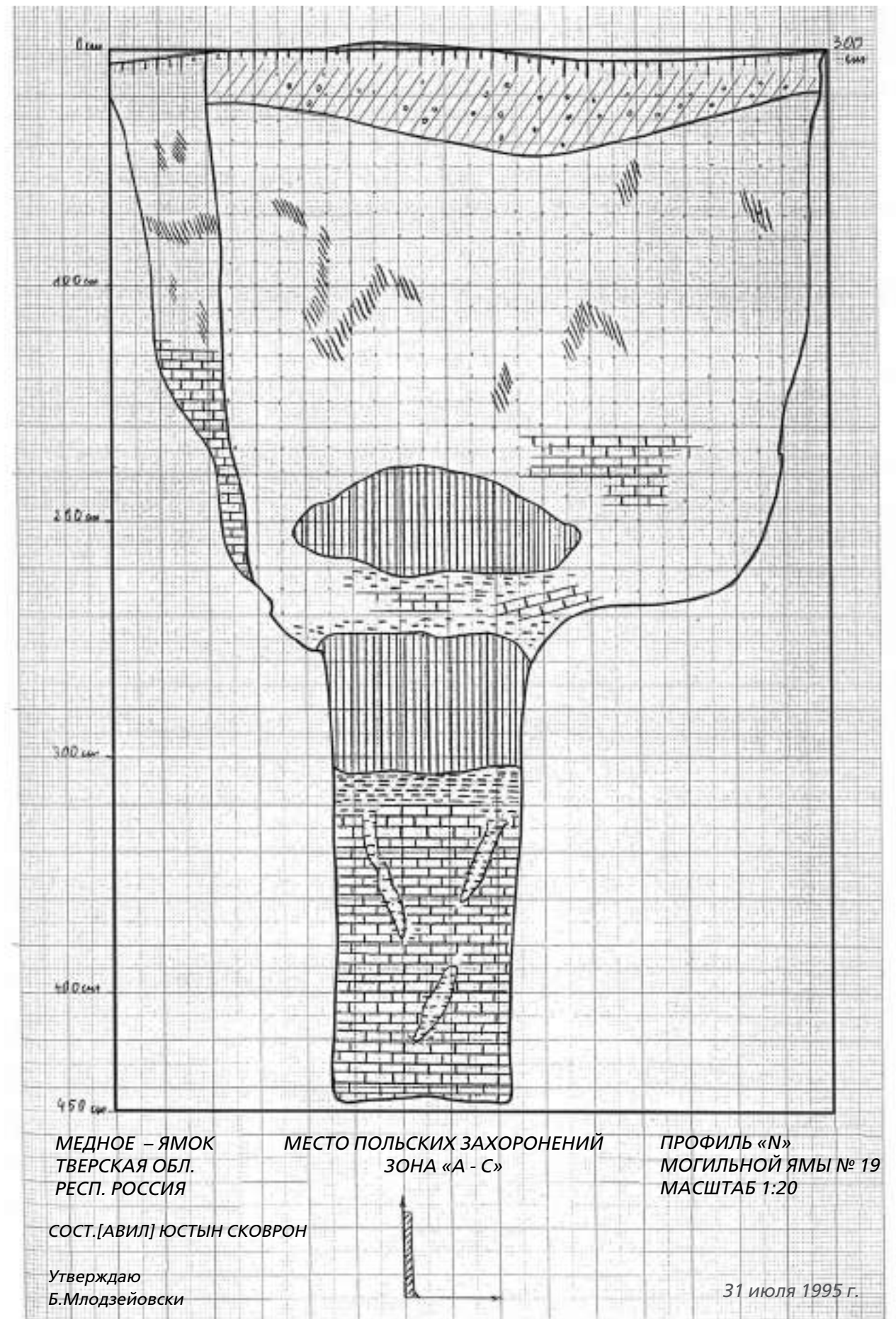
[Геологический профиль могильной ямы № 19. Условные обозначения объяснены на последней странице тома III отчета (см. ниже с. 650)]
